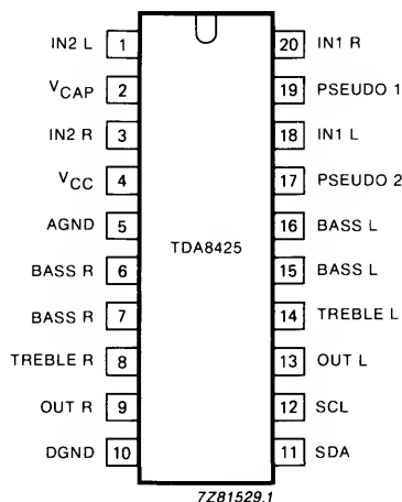
Fig. 2 Pinning diagram.
