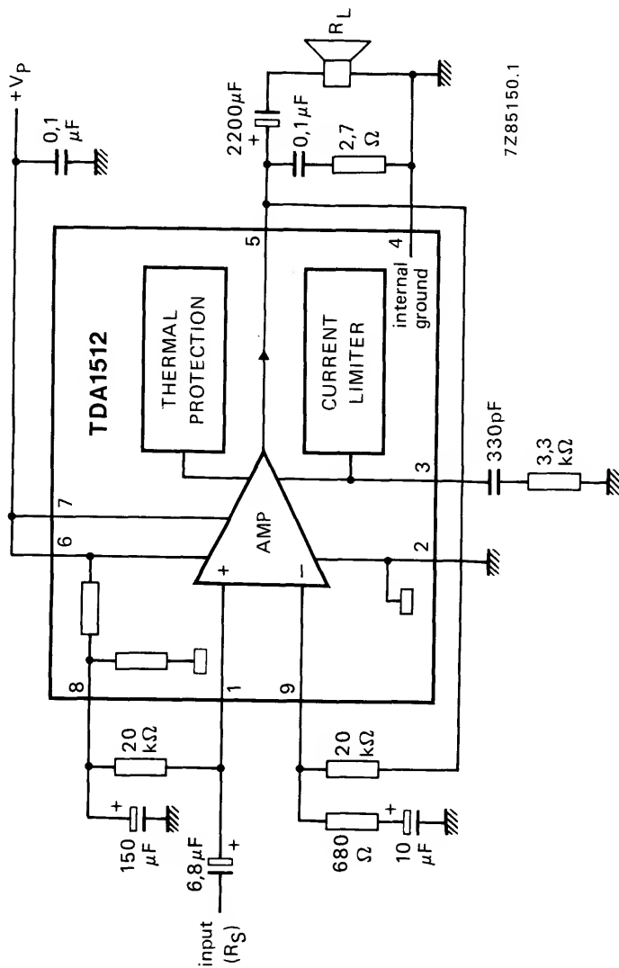
Fig. 3 Test circuit.
