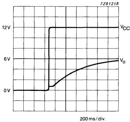
Fig. 18 Turn-on behaviour; C = 2,2 \mu F ; R_L = 10 \text{ k}\Omega .
