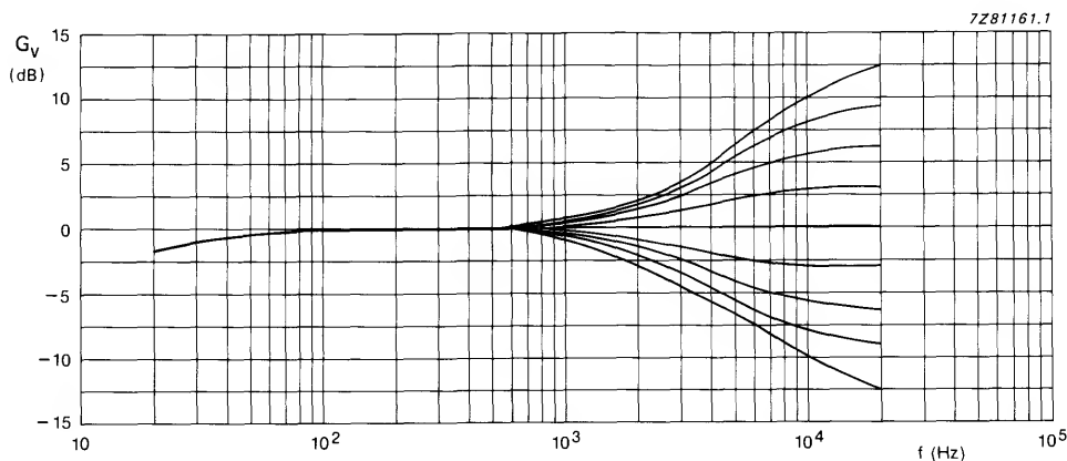
Fig. 6 Treble control.
