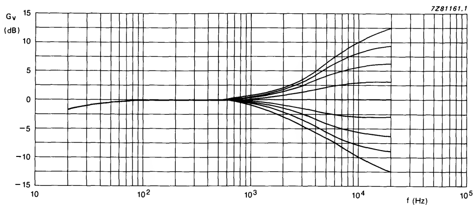
Fig. 6 Treble control.
