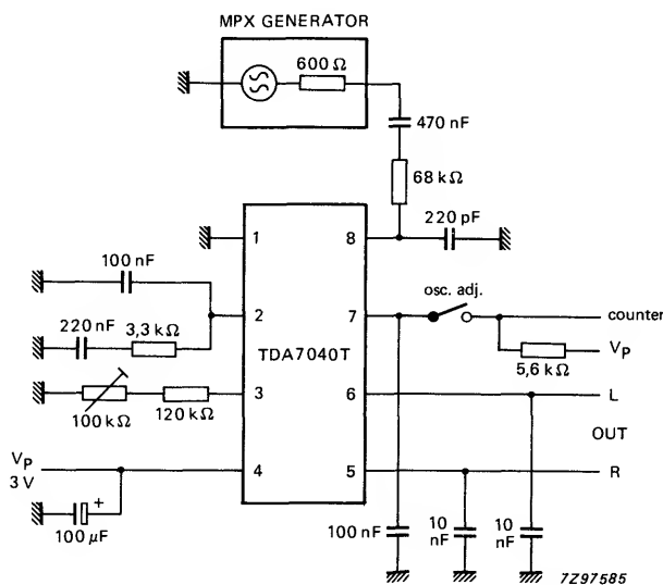
Fig. 2 Test circuit.
